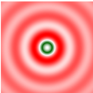
Sinus cardinal
