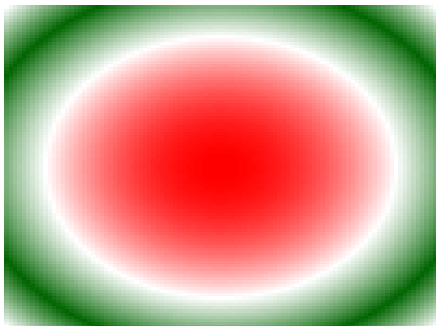
Sinus cardinal
